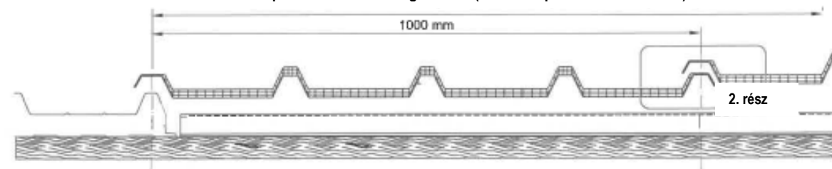
több CUTA 5 panelből készült világítóablak (1000 mm*panelek N* számával)
