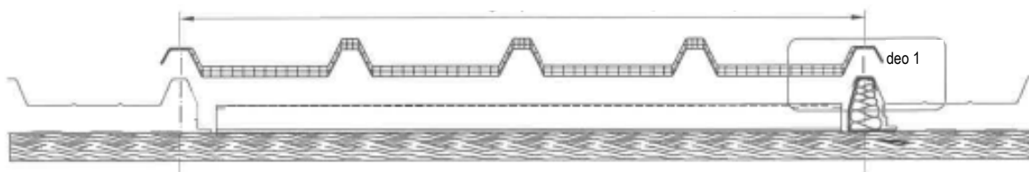
Prozor od više panela CUTA 5 (1000 mm *N* panela)
