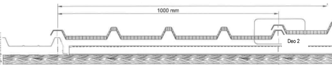
Više preklopljenih ploča CUTA 5 (1000 mm *N*panela)
