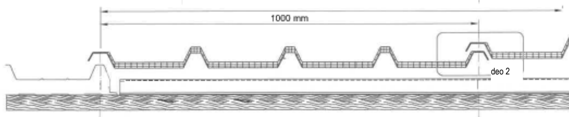
Prozor od više panela CUTA 5 (1000 mm *N* panela)
